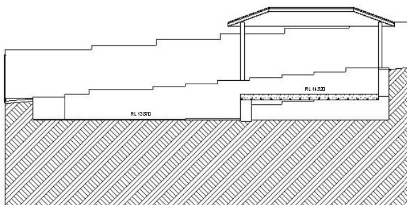
SECTION A2
